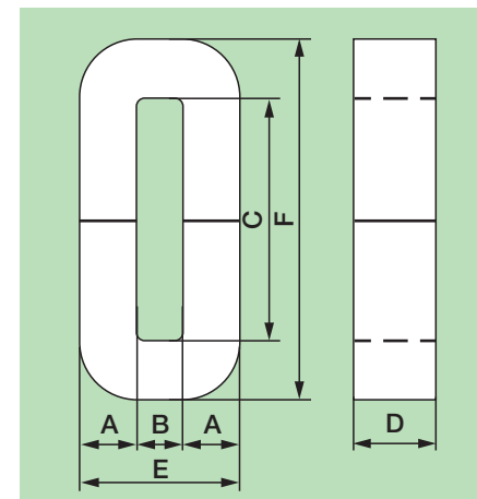
Fig 2. Shape of cut core 図2. カットコアの形状
